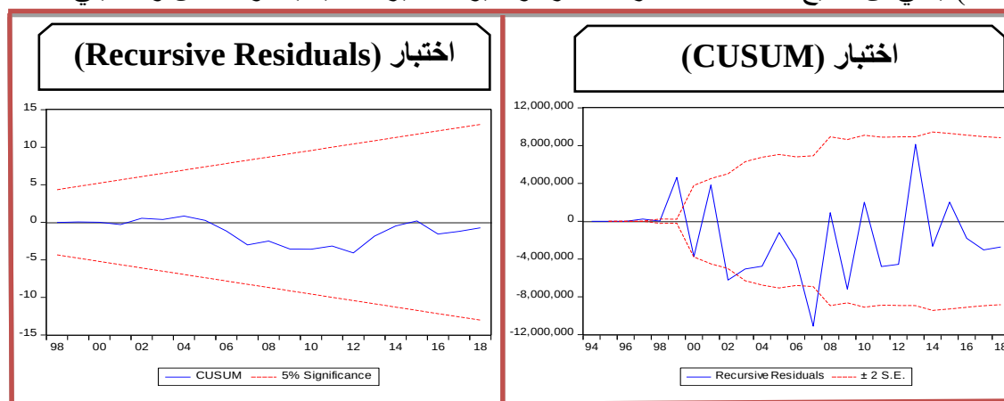
الشكل (4): نتائج اختبار استقراريه الانموذج المقدر لدالة الانفاق الاستثماري
