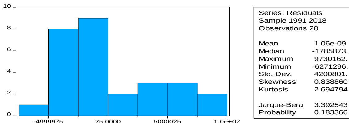
الشكل (3): نتائج اختبار مشكلة التوزيع الطبيعي لأنموذج الانفاق الاستثماري
